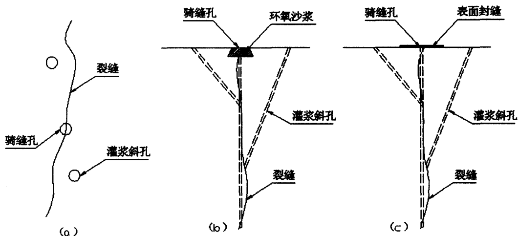
图3 灌浆孔布置示意图
